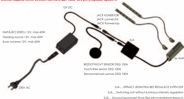
SCHEMA ZAPOJENÍ BEZDOTYKOVÉHO SENZORU BEZ REGULACE SVÍTIVOSTI Connection diagram for touch-free sensor with luminous intensity regulation Схема подключения бесконтактного датчика, без регулировки яркости
